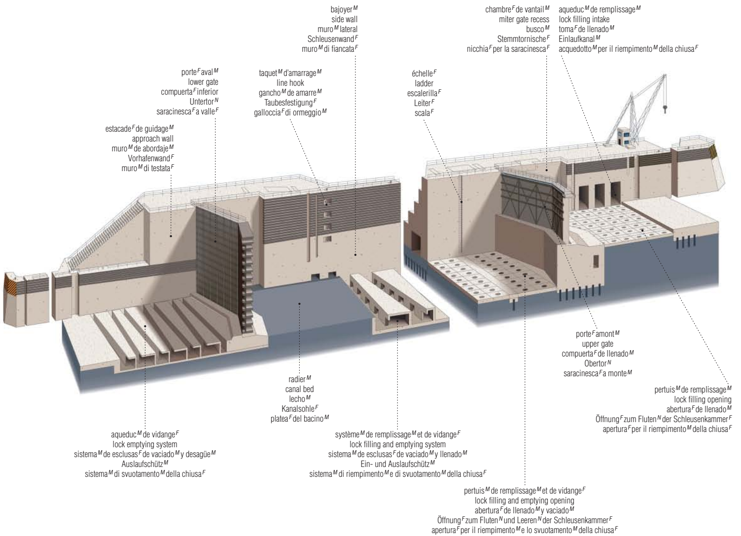
écluse F : vue F latérale canal lock: side view esclusa F : vista F lateral Kanalschleuse F : Seitenansicht F chiusa F di un canale M : vista F laterale
